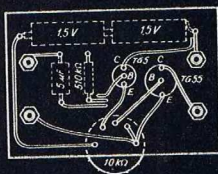
Rys. 2 Schemat montażowy wzmacniacza i wyprowadzenia elektrod tranzystorów
